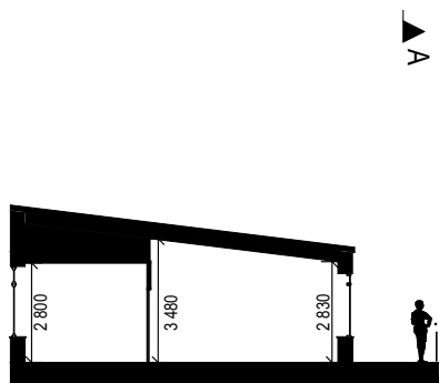
Sektion A-A, Skala 1:200
