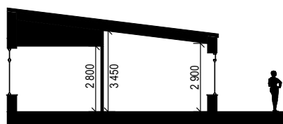
Sektion A-A, Skala 1:200
