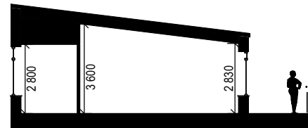
Sektion A-A, Skala 1:200
