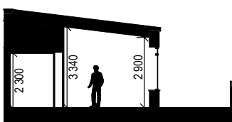
Sektion B-B, Skala 1:200
